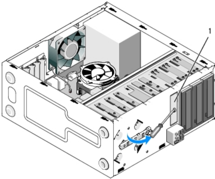
1 herausbrechbare 3,5-Zoll-Metallplatte
