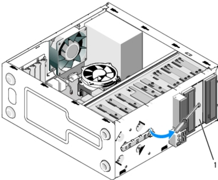
1 5,25-Zoll-Metallplatte (für leeren Schacht eines optischen Laufwerks)
